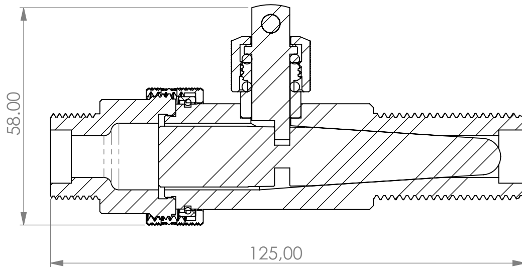
A-A (1 : 1)
